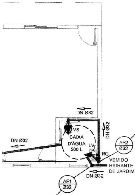
10 PLANTA DE HIDRÁULICA ESCALA 1:100
