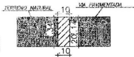
Detalhe do Meio-Fio Rebaixado Sem escala
