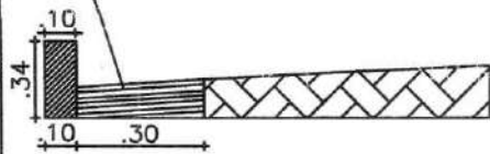
Detalhe da Sarjeta Sem escala
