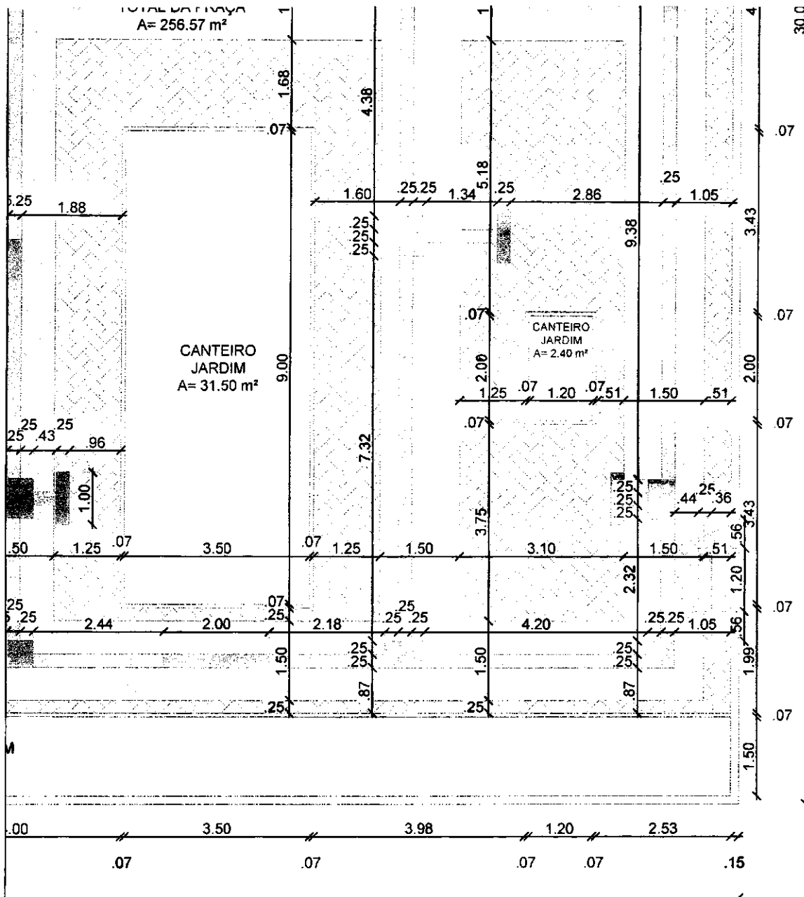
2 PLANTA DE PISO ESCALA 1:100
