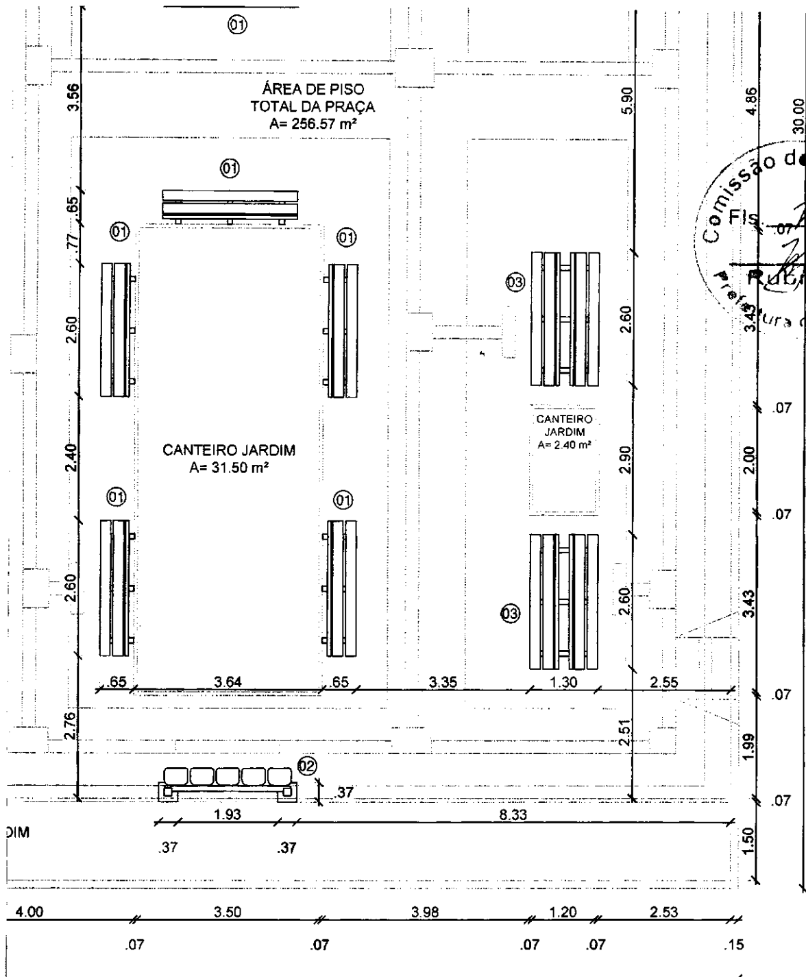
2 PLANTA DE MOBILIÁRIO ESCALA 1:100
